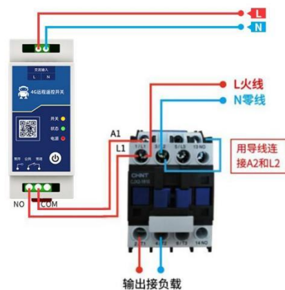
接220V接触器接线图(经典版)
