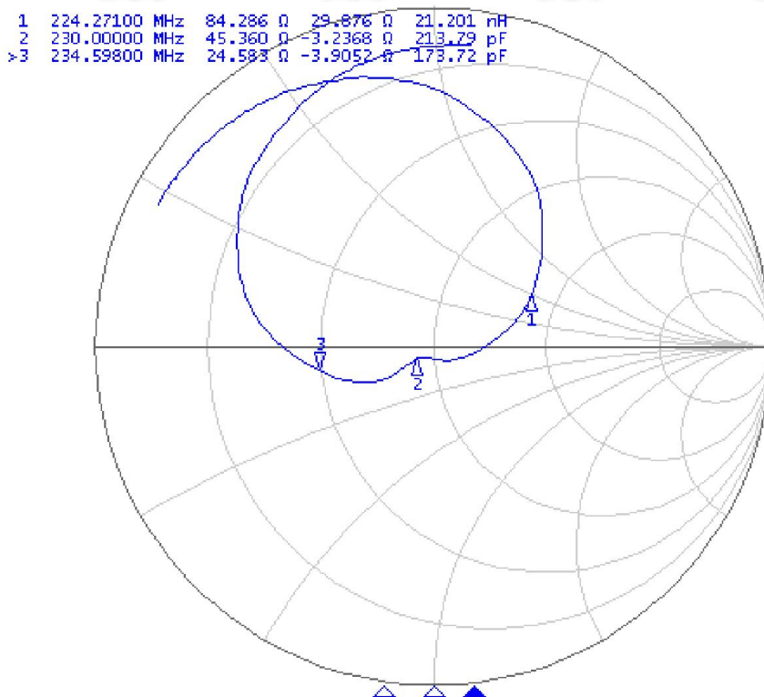
史密斯圆图 (Smith chart)
