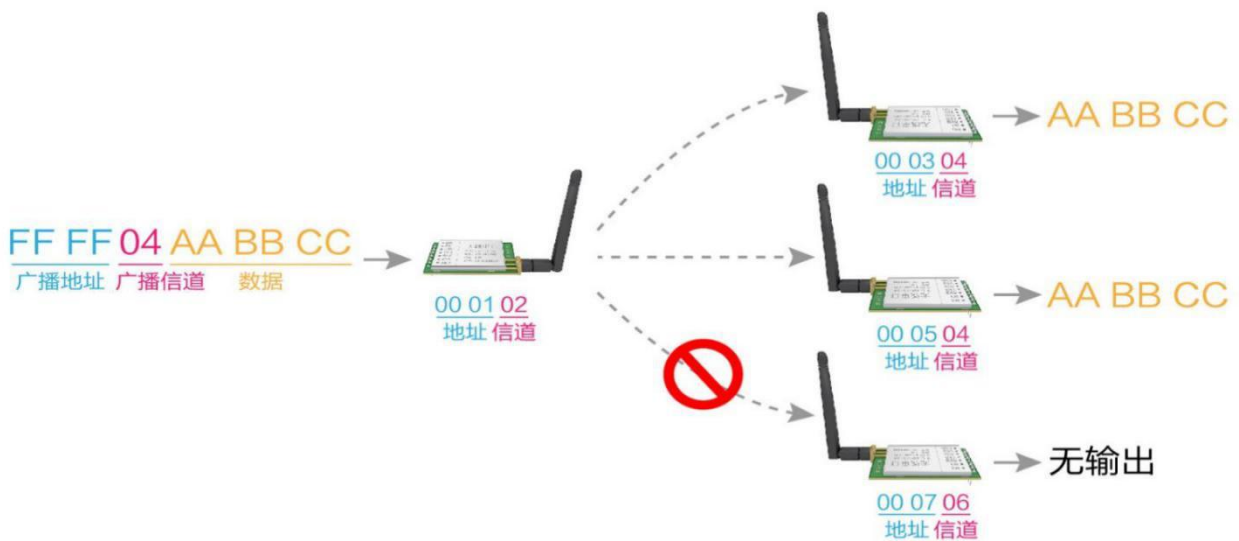
图 5-2 广播发射
