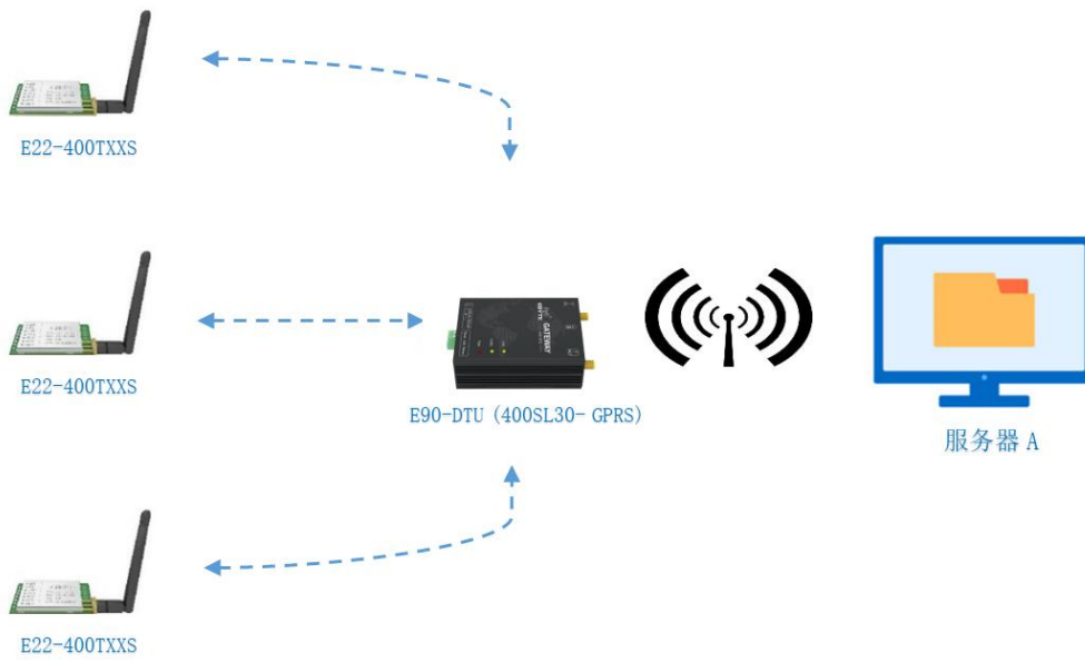
( 2 ) E90-DTU(400SLxx) + E90-DTU(400SL30- GPRS) + 服务器 A
