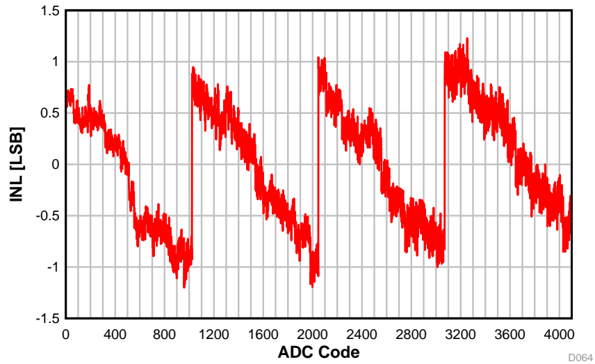
图 5-51. INL vs. ADC Code
