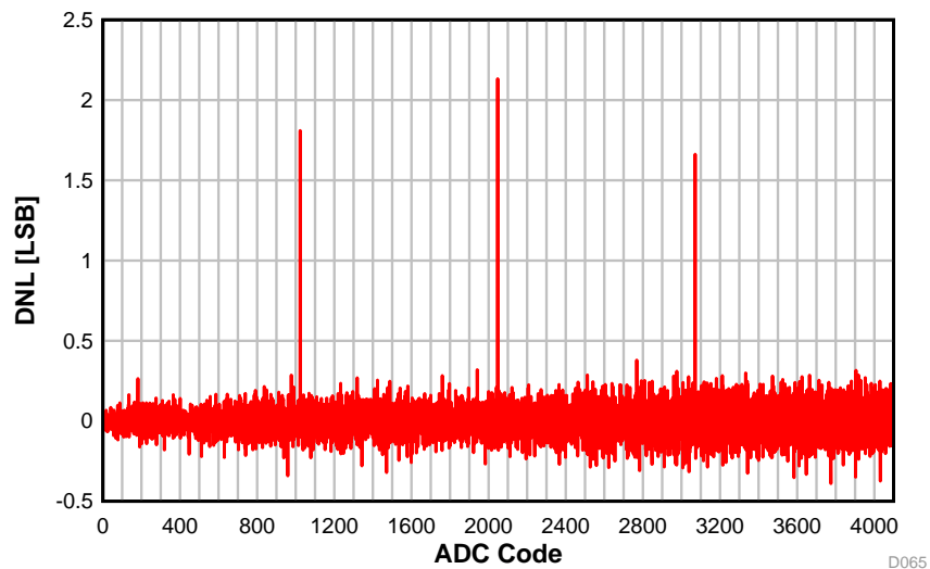
图 5-52. DNL vs. ADC Code
