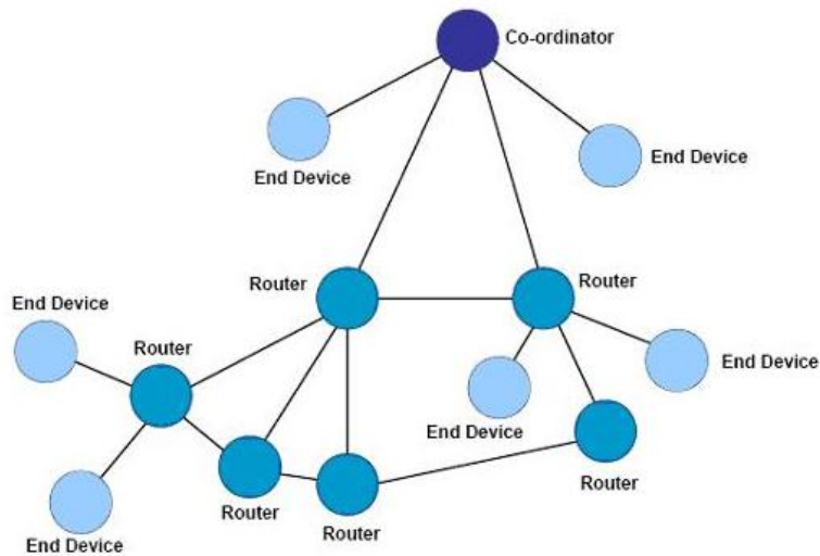
网络结构图
