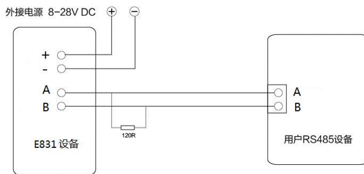
RS485接线图
